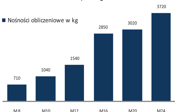
Nośności obliczeniowe na wrywanie prętów gwintowanych TCS klasa stali 5.8 z betonu C20/25 w kg
